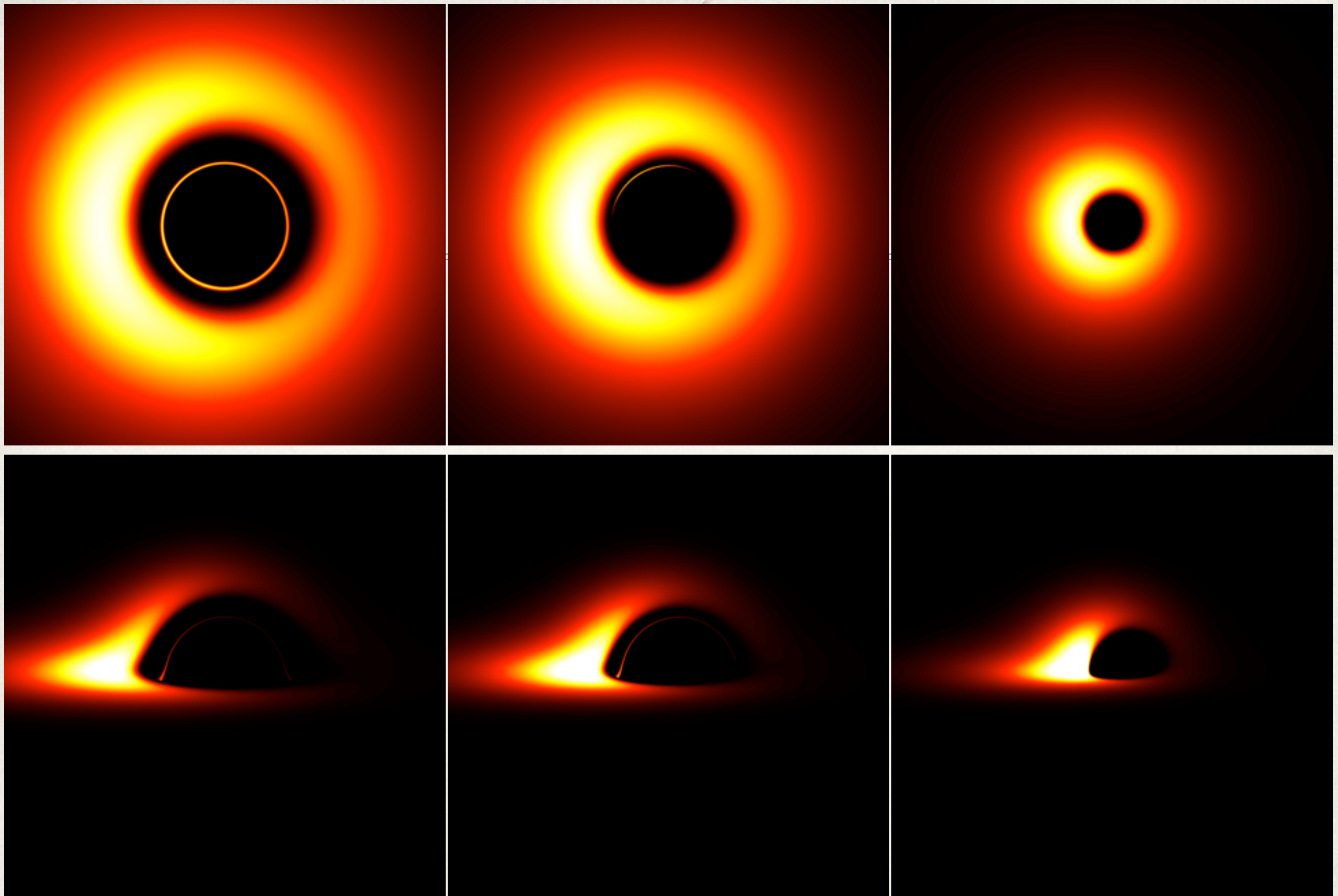
光学的に厚く幾何学的に薄いブラックホール降着流のイメージ Kerrブラックホールの スピン(回転の度合いを表す): a^* = 0, 0.5, 0.999 (左図から右図), 観測者が見る位置: i = 10^\circ (上の図), 85^\circ (下の図), これらは一般相対論的輻射輸送計算により計算した。
