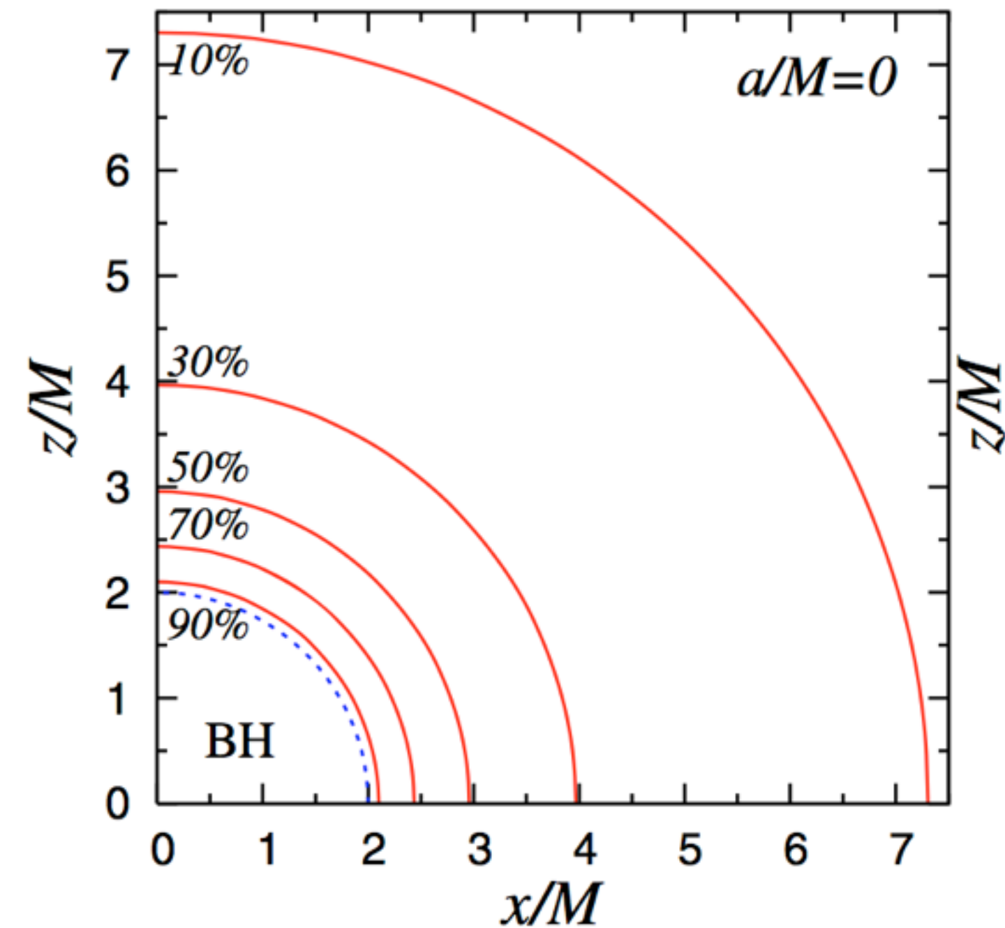
シュバルツシルト・ブラックホールの場合
