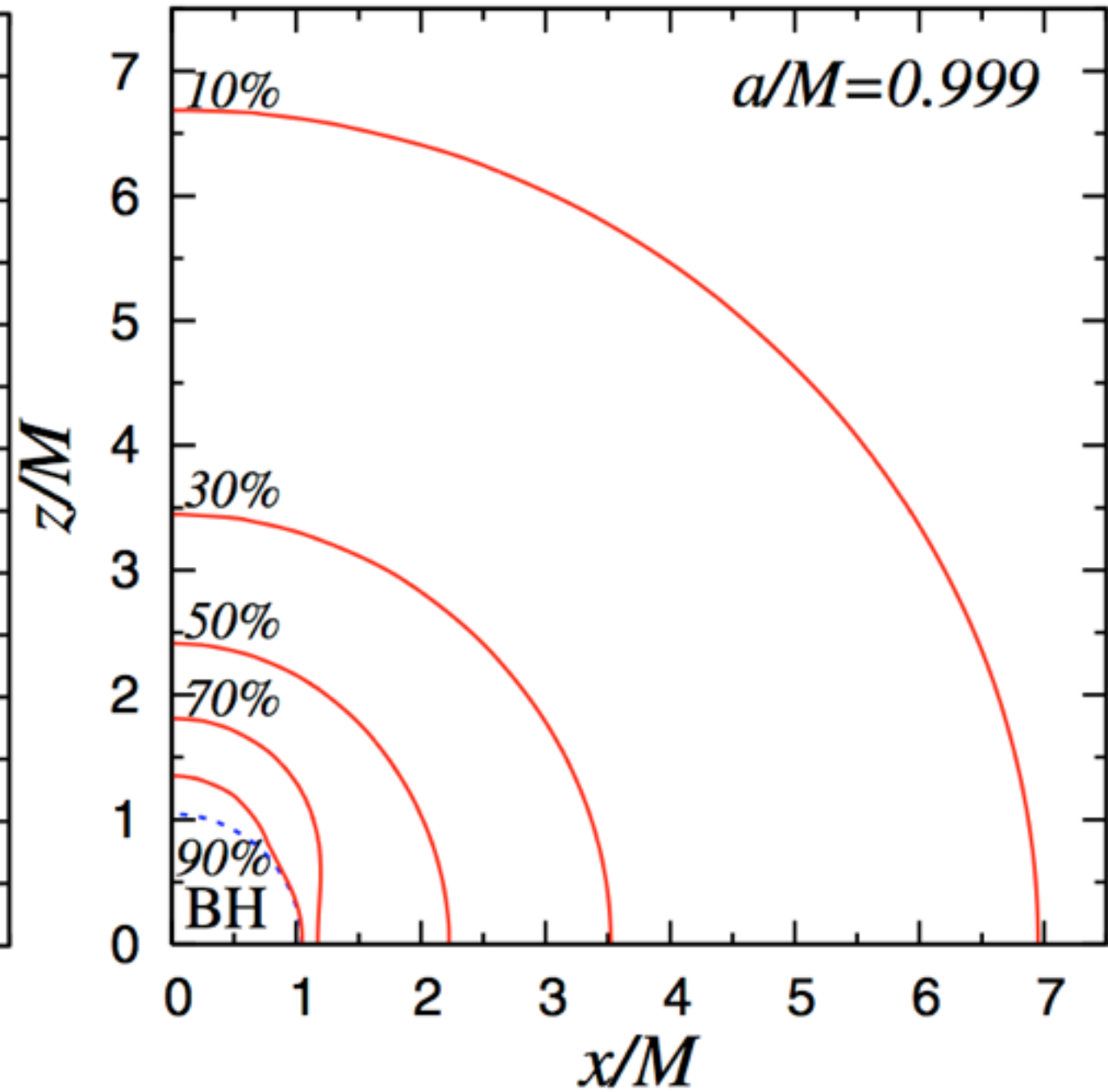
カー・ブラックホールの場合
