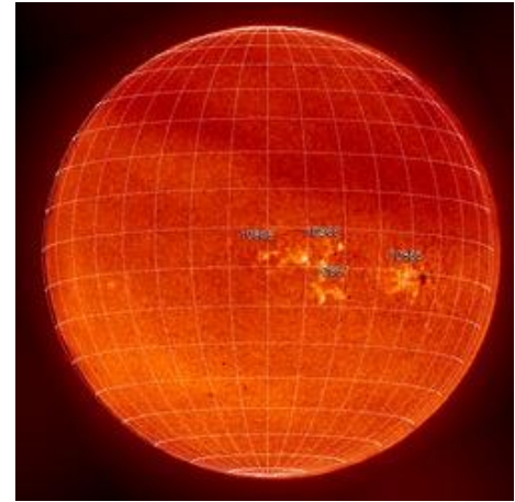
水素H \alpha 線(彩層)
