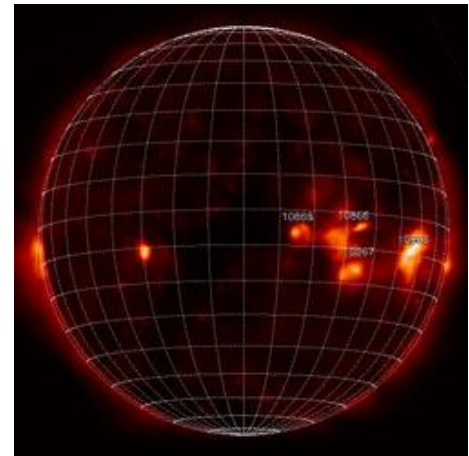
X線(コロナ)
