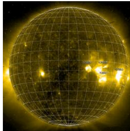
極紫外線(200万度)
